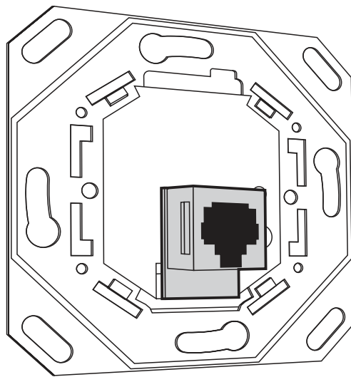
Rys. 1. Prawidłowe podłączenie adaptera do portu magistralnego.
