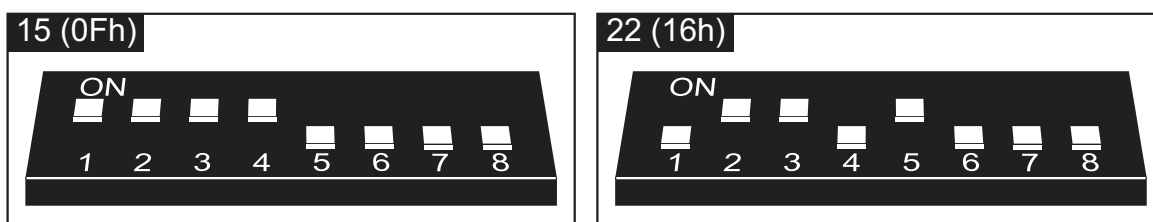
Rys. 2. Przykłady ustawienia adresu (adres 15 (0Fh) wymagany jest przy współpracy z centralami z serii VERSA).
