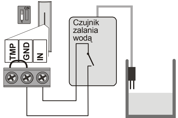
Przykład zastosowania styku NO
