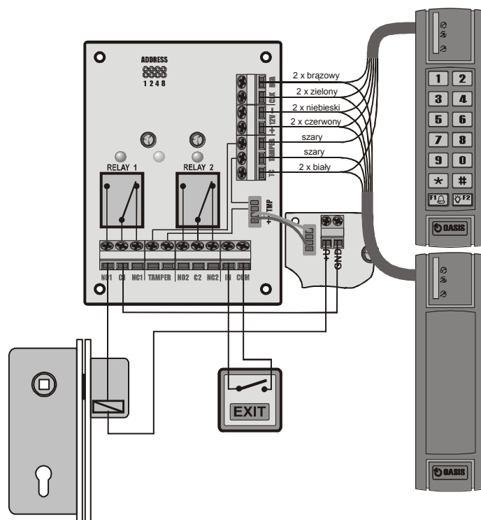
Przykład podłączenia
